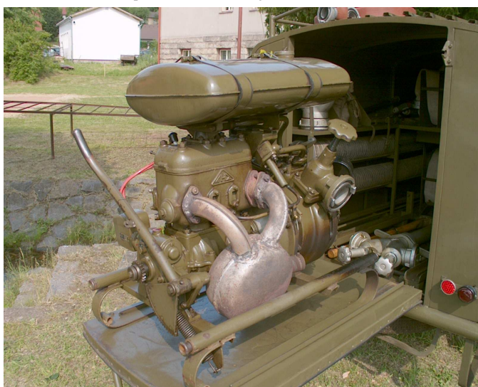
Lhotecká PPS-8 (pojízdňá požární stříkačka)
