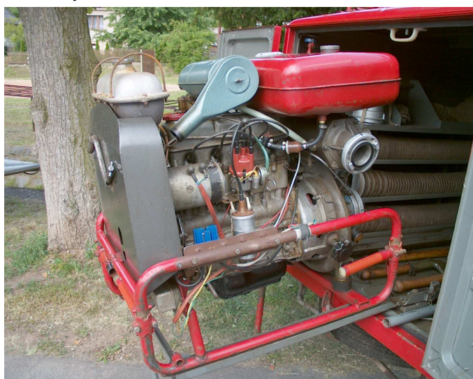
Lhotecká PPS-8 (pojízdňá požární stříkačka)
