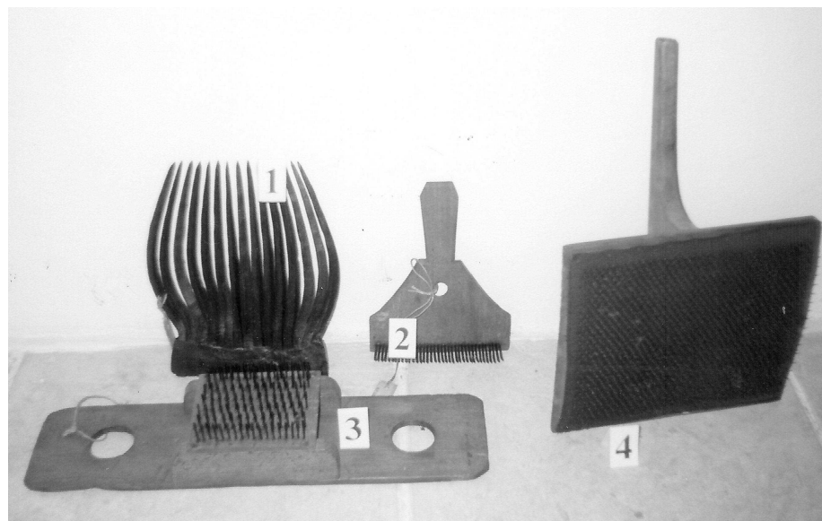
Původní nástroje na domácí zpracování lnu 1. Drhlen, 2. Kracle, 3. Vochle, 4. Vochlice. Vochle se mohla vkládat do tzv. vochlovací stolice (podle potřebné hustoty kartáčů), na které vyčesávač seděl. (Ze sbírek Skanzenu Zubrnice)
